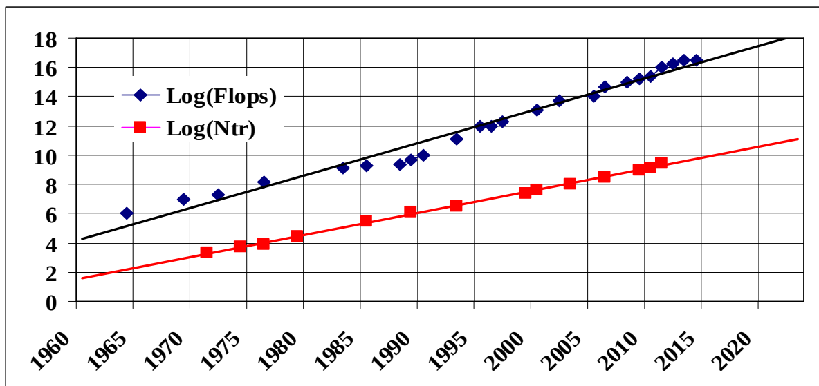
Рис. 9.2. Закон Мура и производительности суперкомпьютеров (в флопсах)
