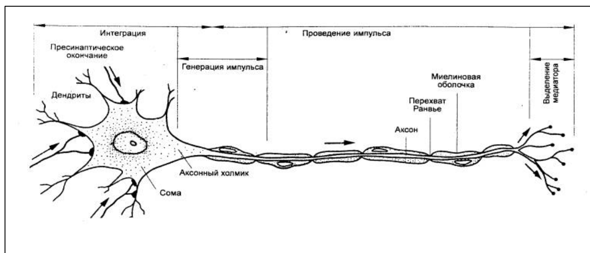
Рис. 6.3. Схема нейрона
